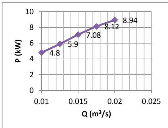
Gambar 4.2 Grafik pengaruh debit (Q) terhadap daya (P) pada data hasil penelitian
