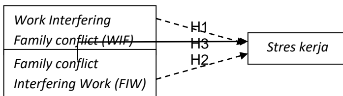
Gambar 1. Kerangka Penelitian
