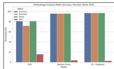
Gambar 3.1 Grafik Perbandingan Kinerja Model
