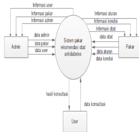
Gambar 2. Diagram konteks sistem rekomendasi obat
