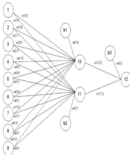
Gambar 4. Arsitektur Jaringan Saraf Tiruan Backpropagation Fertilitas
