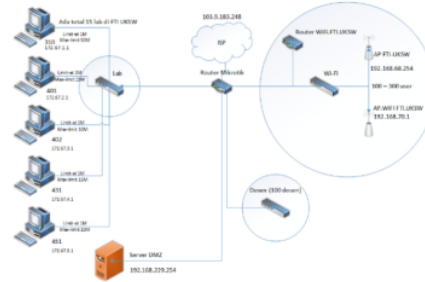
Gambar 3. Topologi jaringan sesudah dilakukan perancangan HTB
