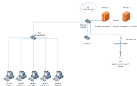
Gambar 2. Topologi sebelum dilakukan perancangan HTB
