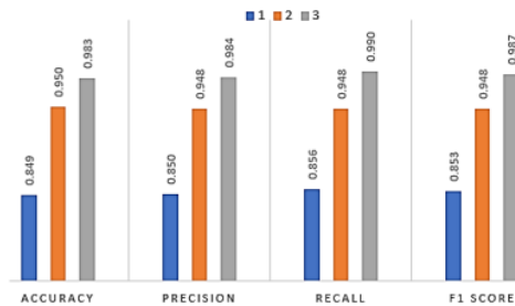
Gambar 7. Hasil pengujian setelah transfer learning
