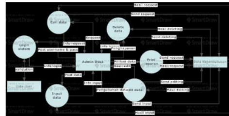
Gambar 2. Perancangan DFD SIDK.
