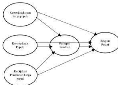
Gambar 1: Model Analisis Jalur
