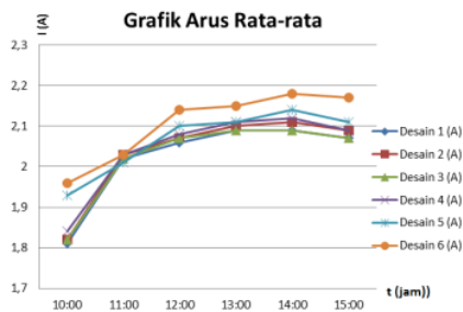
Gambar 4. Grafik Nilai Arus Rata-rata Desain1-6
