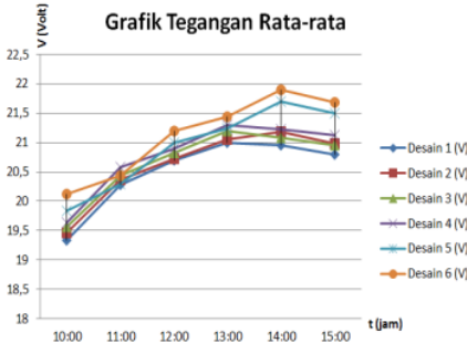
Gambar 5. Grafik Nilai Tegangan rata-rata Desain1-6
