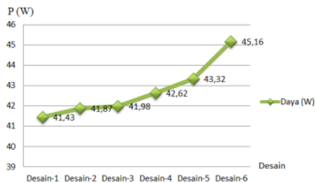
Gambar 6. Grafik Daya keluaran rata-rata Desain 1-6
