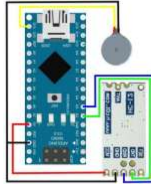
Gambar 11 Gambar Rangkaian Makmum
