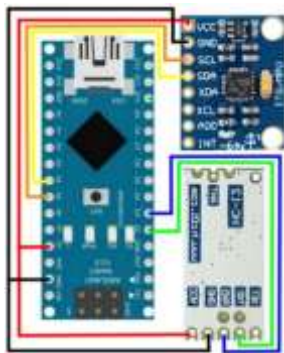
Gambar 10. Rangkaian Perangkat Imam
