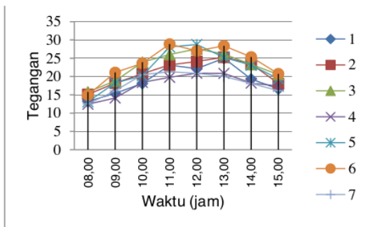
Gambar 2. Grafik Tegangan Solar Cell Secara Keseluruhan
