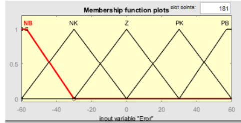
Gambar 11: Fungsi Keanggotaan Error
