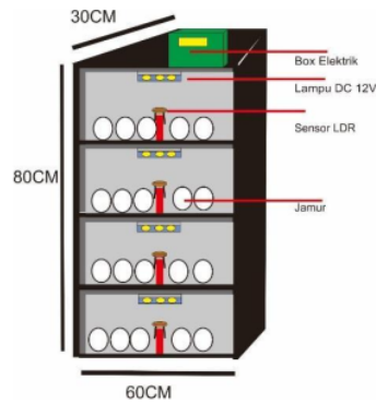
Gambar 4: Perancangan Mekanik
