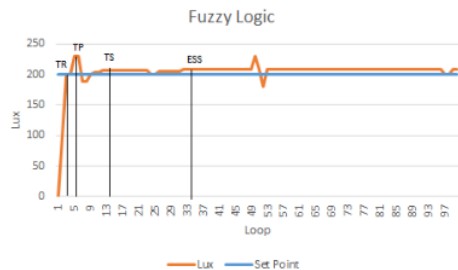
Gambar 17: Grafik Fuzzyfikasi 1
