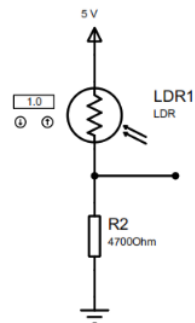
Gambar 7: Rangkaian Pembagi Tegangan LDR
