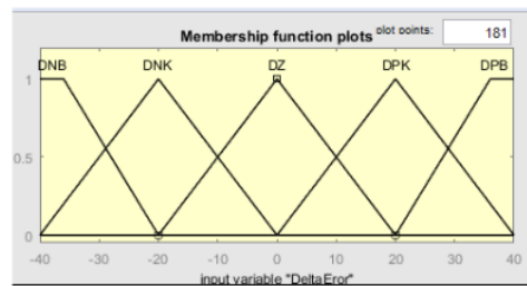
Gambar 12: Fungsi Keanggotaan delta Error
