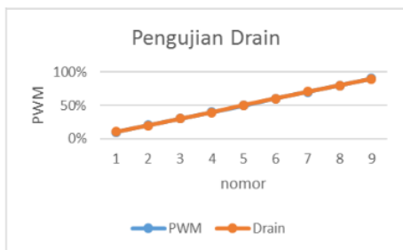
Gambar 15: Grafik pengujian Mosfet kaki drain
