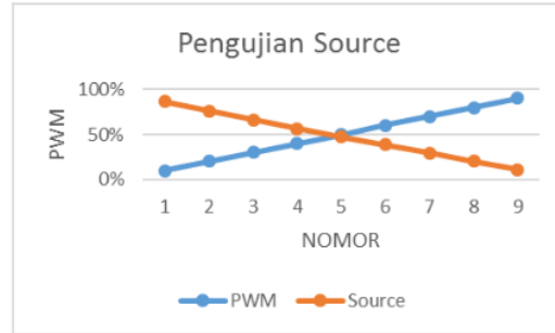
Gambar 16: Grafik pengujian driver Mosfet sisi source
