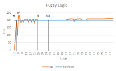
Gambar 18: Grafik Fuzzyfikasi 2
