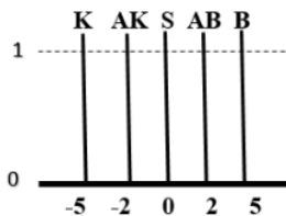
Gambar 13: Fungsi Keanggotaan delta Error
