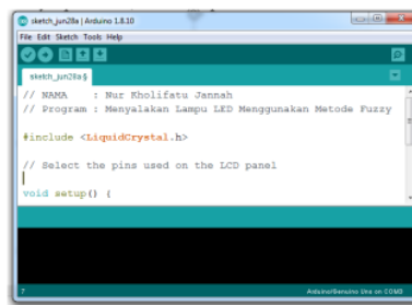
Gambar 3: IDE Arduino
