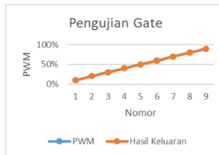
Gambar 14: Grafik pengujian driver Mosfet sisi gate
