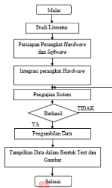
Gambar 7. Kerangka Penelitian
