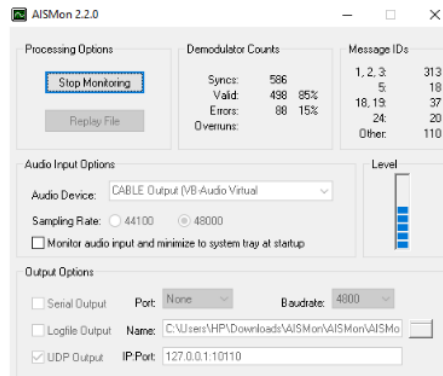
Gambar 16. Hasil Decoding Data
