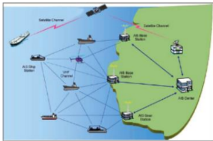
Gambar 1. Skema Komunikasi Data AIS
