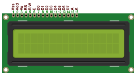
Figure. 5 IC LCD 16x2
