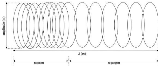
Figure. 2 Longitudinal Waves
