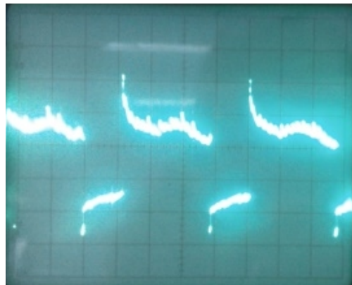
Gambar 10. Sinyal kondisi motor belok kiri
