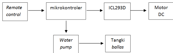
Gambra 6. diagram blog sistem kerja penggerak dan ballas pada mini ROV
