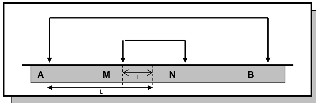
Gambar 1. Susunan Elektroda Metoda Schlumberger
